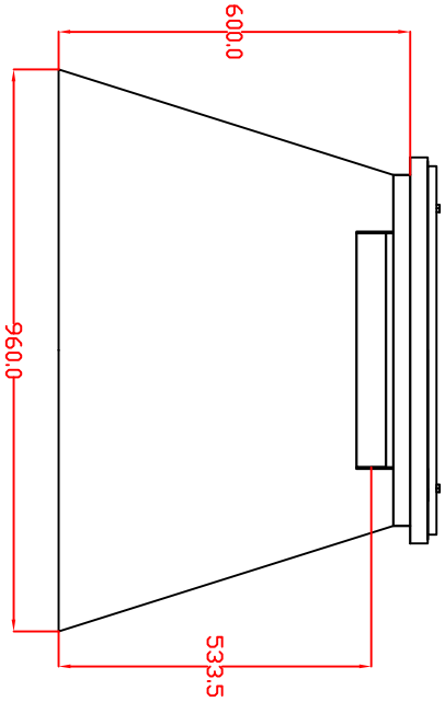
Rain Cover 600T L Artikalnř: 7172063T
