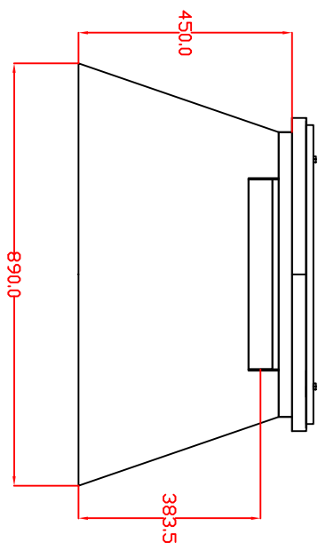
Rain Cover 600T M Artikalnř: 7172063T
